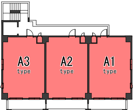
2-7階平面図
