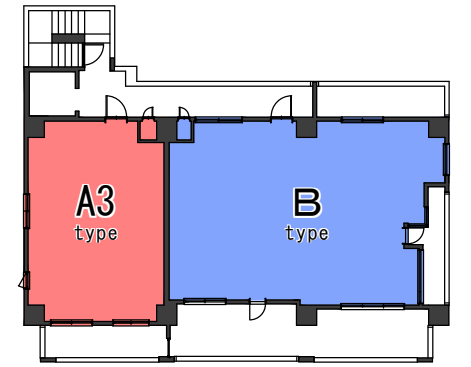
8階平面図
